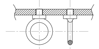
Рыи для подъема орудийного замка М 1:10
