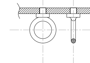
Рыи для подъема орудийного замка М 1:10
