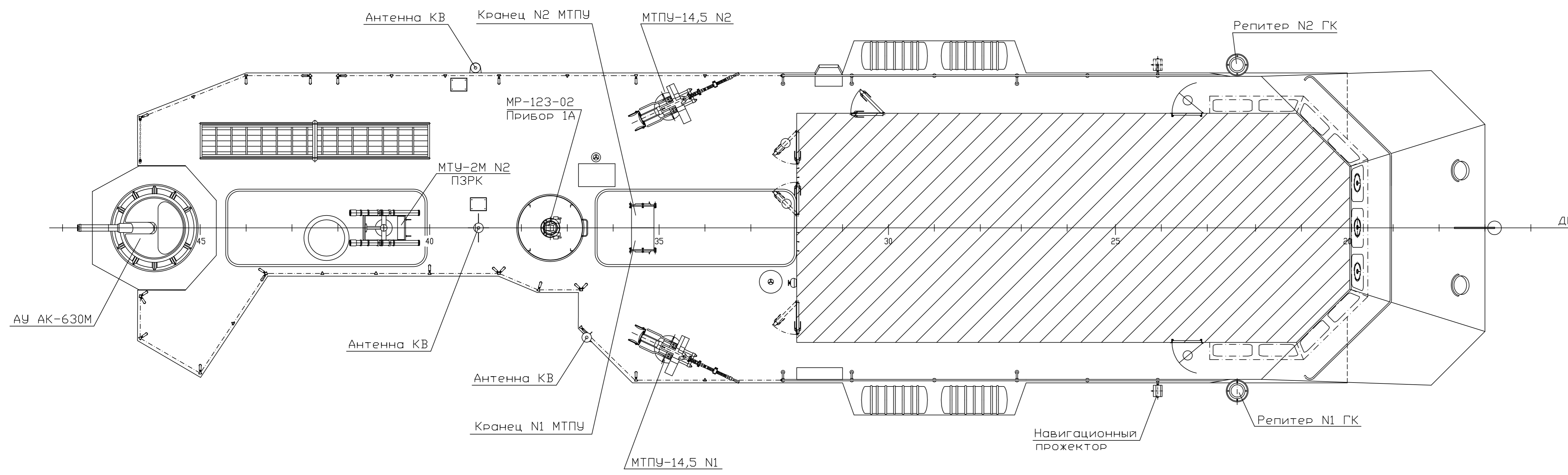
Палуба надстройки 1 яруса
