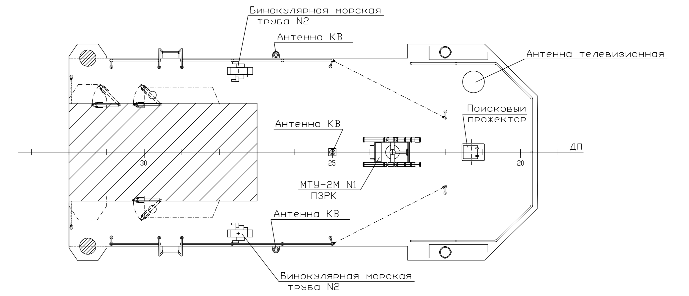
Палуба надстройки 2 яруса
