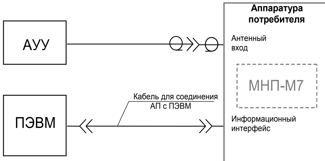
Рисунок 9 – Схема подключения МНП-М7 при работе по реальному сигналу
