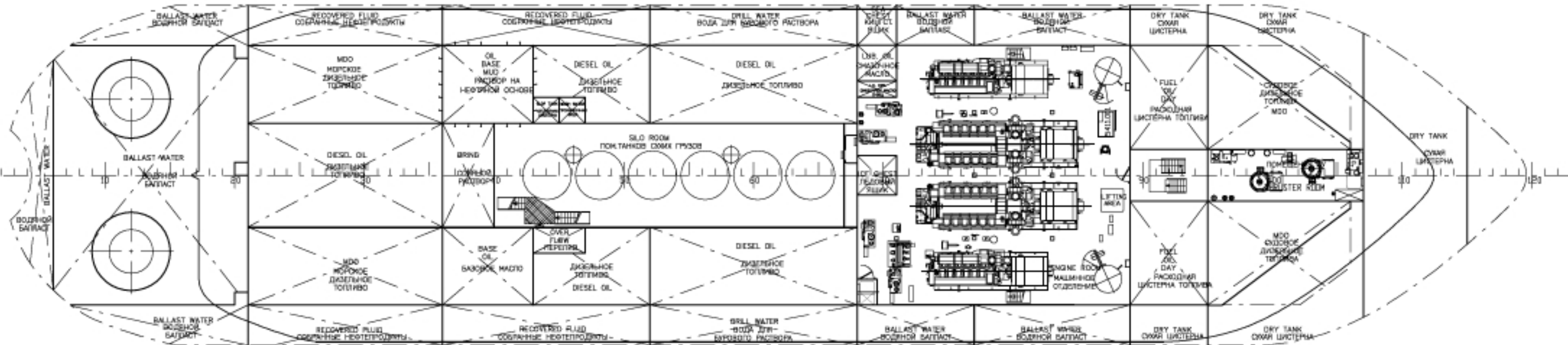
PLATFORM 5100 (Deck 2) С/П № 2 ПЛАТФОРМА 5100 (ПАЛУБА 2)
